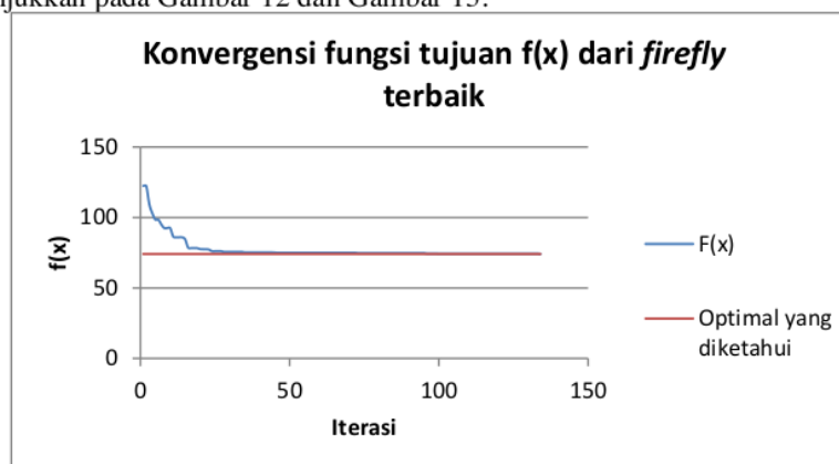
Gambar 12. Grafik fungsi tujuan dari firefly terbaik pada kasus Ulysses16
