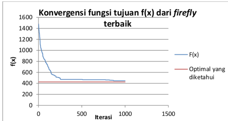
Gambar 13. Grafik fungsi tujuan dari firefly terbaik pada kasus Eil51
