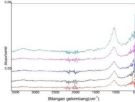
Gambar 1. Spektra FTIR alang-alang sebelum dan setelah pretreatment hidrotermal
