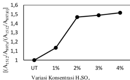
Gambar 2. Pengaruh konsentrasi asam encer terhadap komposisi lignin
