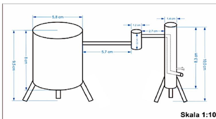
Gambar 1. Desain alat pirolisis yang digunakan.
