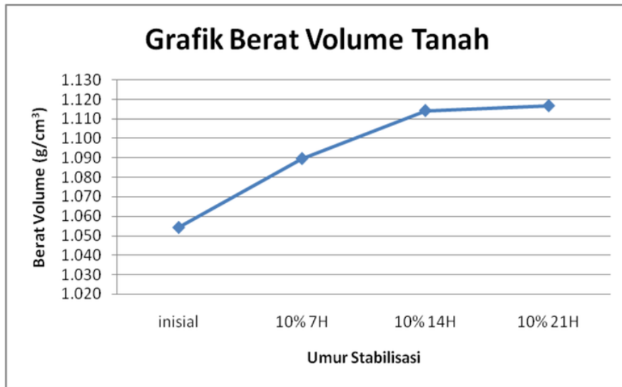
Gambar 2. Grafik hubungan berat volume tanah ( \gamma ) dan masa peram bahan stabilisasi
